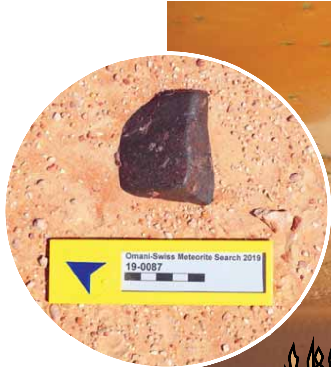
■ إحدى القطع النيزكية التي تم العثور عليها
