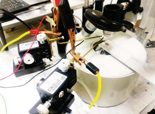
■ جهاز الميكروسكوب المغناطيسي الضوئي لظاهرة كير ( Kerr )
