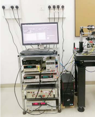
■ جهاز الميكروسكوب المغناطيسي الضوئي لظاهرة كير ( Kerr )
