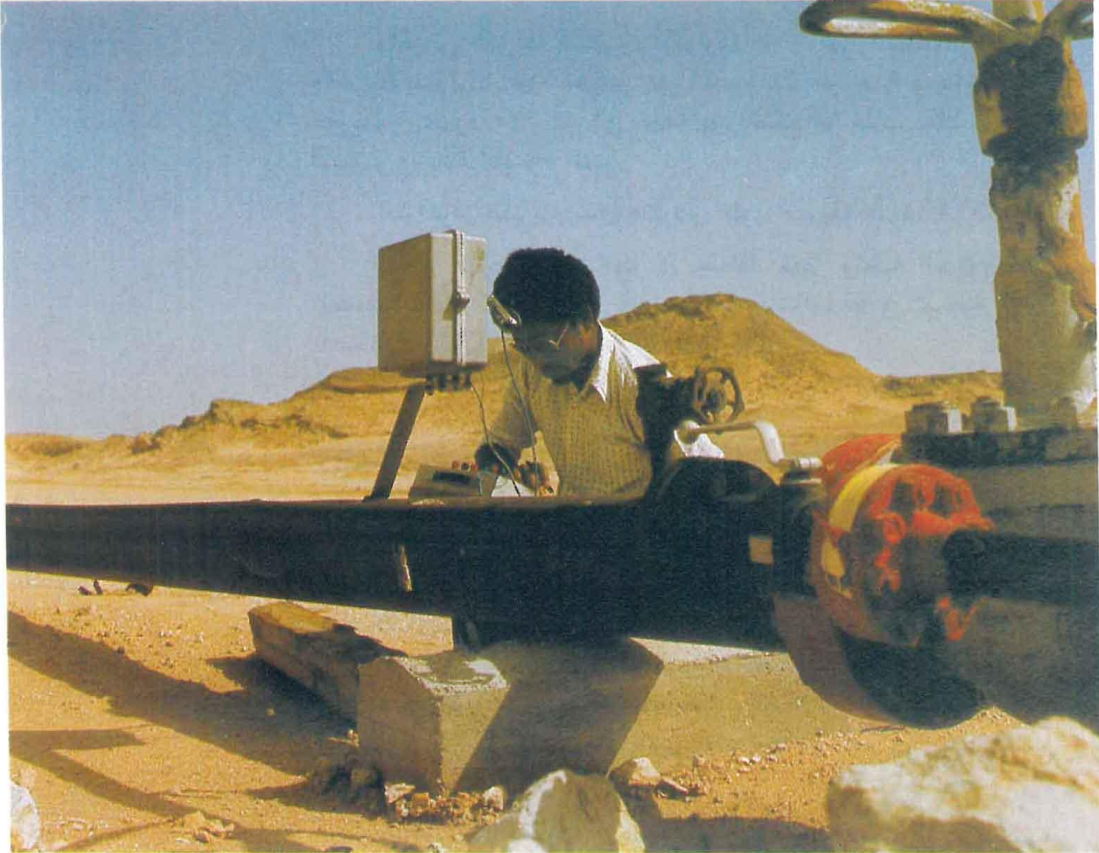
فحص خط أنابيب النفط
