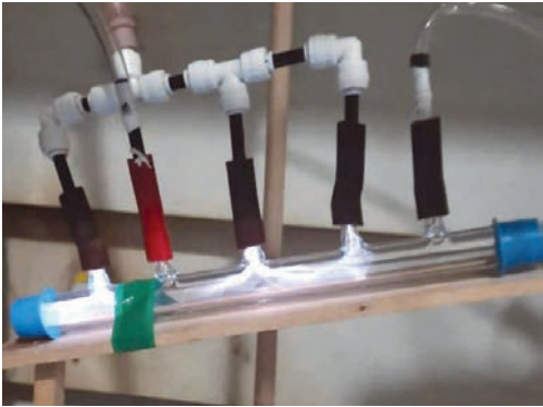
■ مفاعل البلازما اللاحرارية متعدد الشعل النفاثة المطور في مختبرات جامعة نزوى
