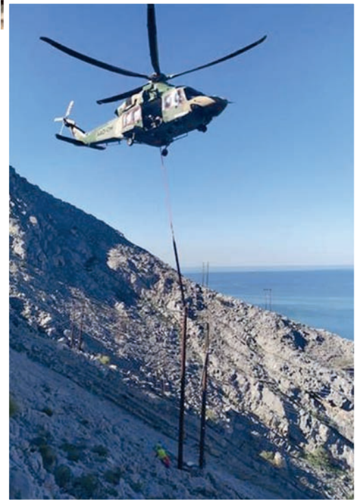
تواجد خطوط النقل الكهربائي بمسارات جبلية تحد كبير يصعب فيها إنجاز الصيانة للأعطال في حال حدوثها.
