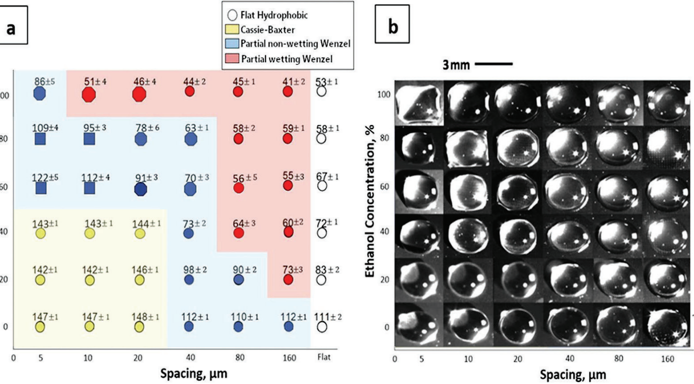
صورة مجهرية للخارطة التكاملية لخواص قطرات الكحوليات والماء ومخاليطهن الثنائية على الأسطح المعدلة هندسياً التي تم نشرها في إحدى المجلات العلمية
