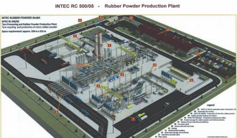
■ مخطط توضيحي لمشروع إعادة تدوير الإطارات
