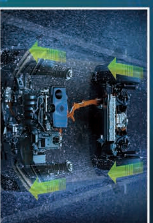
محرك هايبرد من الجيل الخامس سعة ٢,٥ لتر
